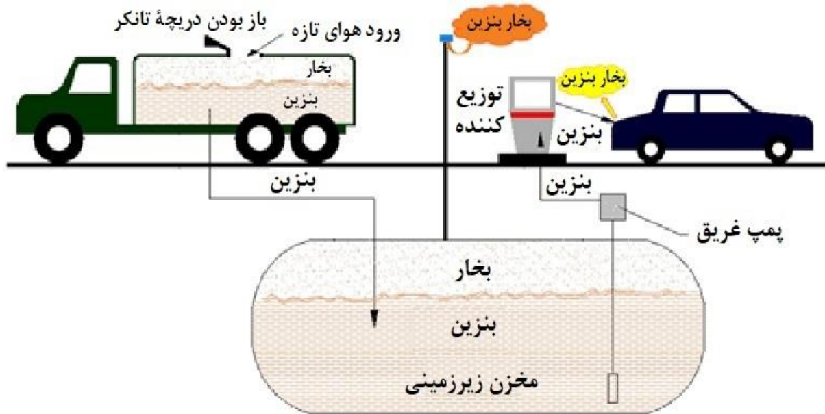
شکل ۱- شماتیک انتشار بخار بنزین حین تخلیه تانکر و سوخت‌گیری خودرو در پمپ بنزین قبل از اجرای طرح کهباب
